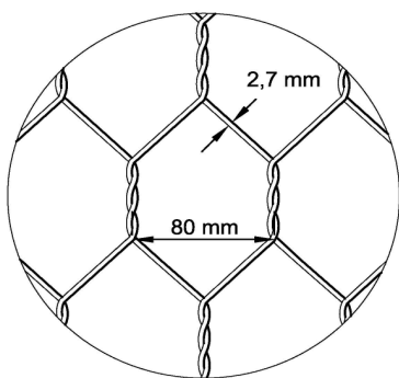
A malha é hexagonal de tripla torção
