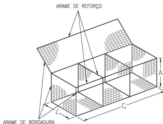
Gabião de 3x1x1 com diafragmas.
